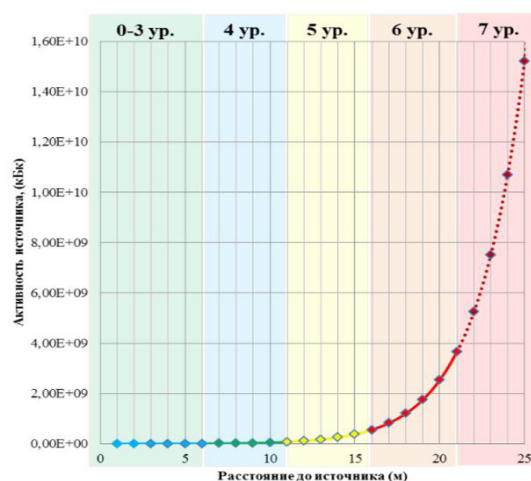
Рис. 5. График зависимости A_{\text{Pu-239}}(X) при D=\text{const}=100 \text{ нЗв/ч}
