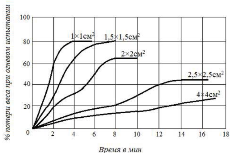
Рис. 3. Изменение скорости горения деревянных брусков от их поперечного сечения
