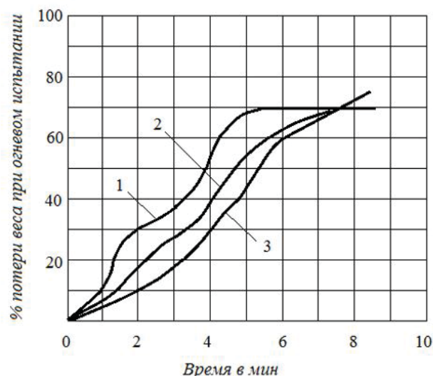
Рис. 2. Изменение скорости горения древесины от плотности: 1 – \rho = 350 \text{ кг/м}^3 ; 2 – \rho = 540 \text{ кг/м}^3 ; 3 – \rho = 620 \text{ кг/м}^3
