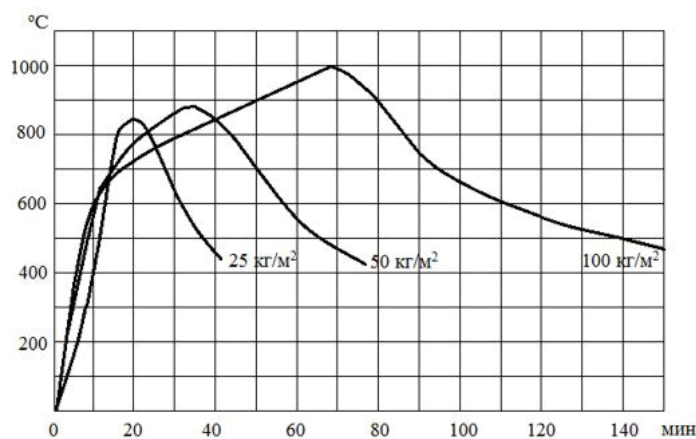
Рис. 4. Температурный режим пожара в зависимости от размещенного на площади количества древесины
