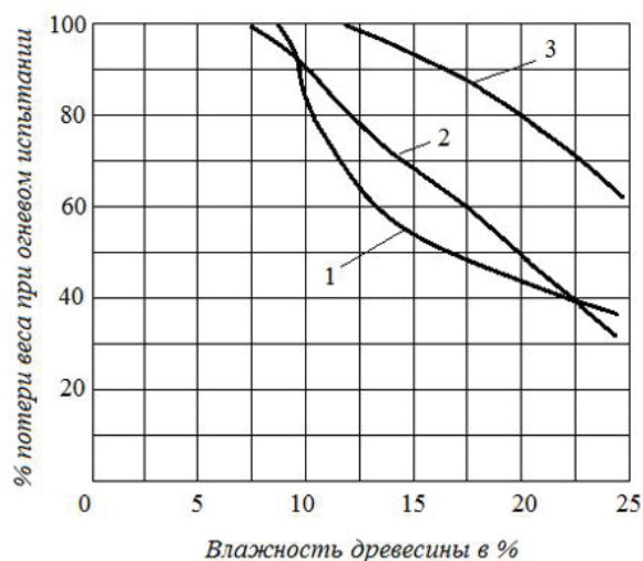
Рис. 1. Изменение скорости горения древесины от влажности: 1 – ель ( \rho = 550 \text{ кг/м}^3 ); 2 – дуб ( \rho = 770 \text{ кг/м}^3 ); 3 – бук ( \rho = 720 \text{ кг/м}^3 )
