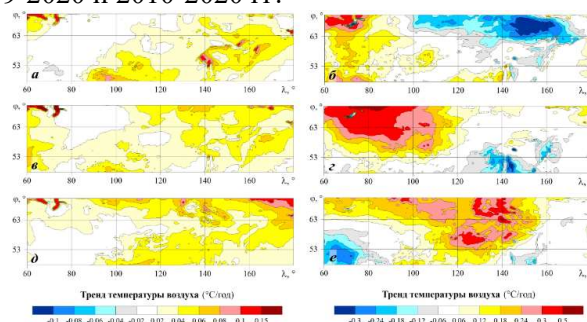
Рис. 5. распределения по территории Сибири значений УКЛТ рядов СТВ для месяцев июль-сентябрь, которые оценены за периоды времени: а) июль 1979-2020гг.; б) июль 2010-2020 гг.; в) август 1979-2020 гг.; г) август 2010-2020 гг.; д) сентябрь 1979-2020 гг.; е) сентябрь 2010-2020 гг.
