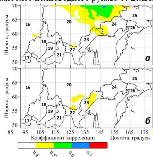
Рис. 3. Участки территории Восточной Сибири, где межгодовые изменения среднемесячных температур воздуха в апреле и мае 1993-2019 гг., были значимо связаны с вариациями S_{СПП} моря Лаптевых для месяцев: а) Май; б) Июнь
