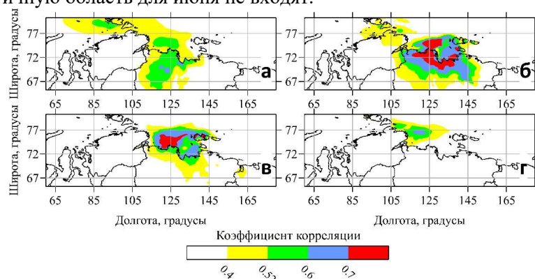
Рис. 2. Участки земной поверхности Арктической зоны Сибири, где связи межгодовых изменений в 1993-2020 гг. СТВ на высоте 2м над ними, а также синхронных вариаций доз ССР, поглощенной всеми льдинами моря Лаптевых, значимы для месяцев: а) Май; б) Июнь; в) Июль; г) Август
