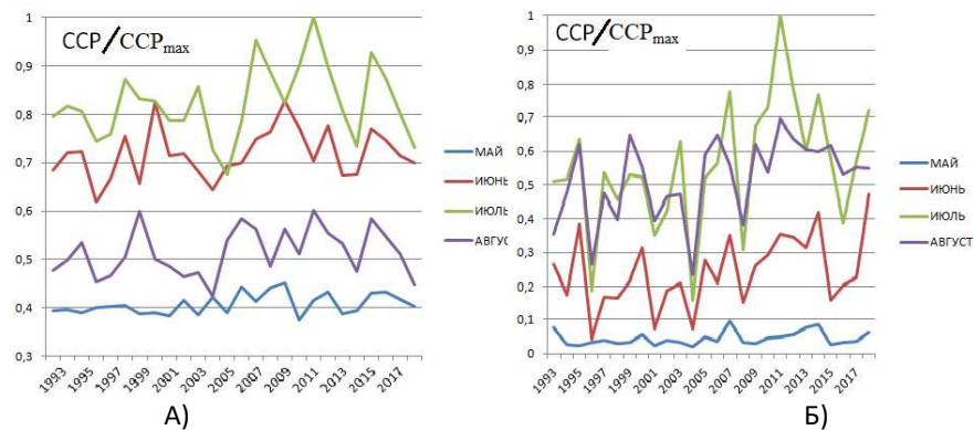
Рис. 1. Зависимости от времени доз ССР для всей акватории моря Лаптевых, нормированных к их максимальным значениям ( ССР_{max} ) за 1993-2019 гг., которые соответствуют месяцам май – август А) падающая; Б) поглощенная
