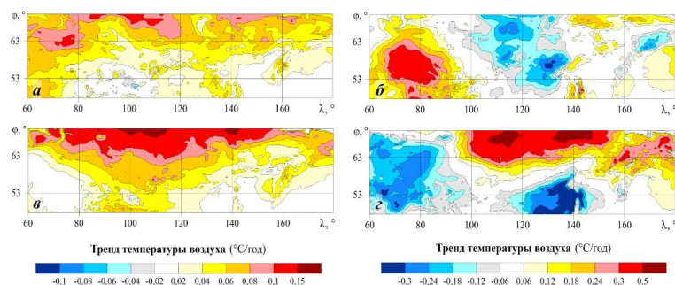
Рис. 4. Распределения по территории Сибири значений УКЛТ временных рядов СТВ на высоте 2м над различными пунктами земной поверхности, для месяцев: а) май 1979-2020; б) май 2010-2020; в) июнь 1979-2020; г) июнь 2010-2020
