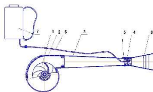
Рис. 3. Устройство для прокладки пенных опорных полос 1-вентилятор, 2- кожух, 3- ствол 4- эжектор, 5 – трубопровод, 6- шланг, 7- ранец- резервуар, 8- пеногенератор
