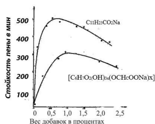
Рис. 2. Влияние солей высших карбоновых кислот на стойкость пены
