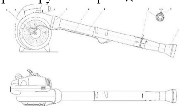
Рис. 4. Устройство для тушения низового лесного пожара 1-вентилятор, 2- кожух, 3- ствол, 4- насос, 5- привод, 6- шланг, 7- пеногенератор, 8- затвор сегментный, 9- привод затвора
