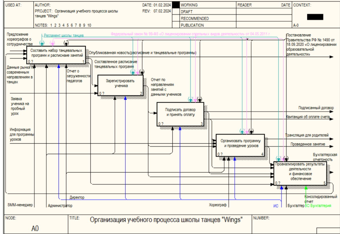
Рис.4. Бизнес-процессы верхнего уровня
