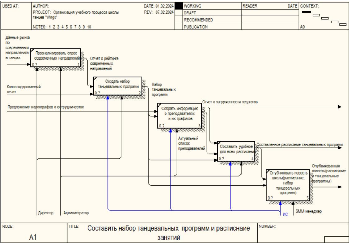
Рис.5. Декомпозиция подпроцесса «Составить набор танцевальных программ и расписание занятий»
