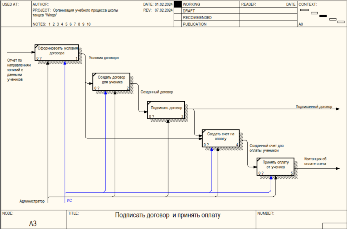
Рис.7. Декомпозиция подпроцесса «Подписать договор и произвести оплату»
