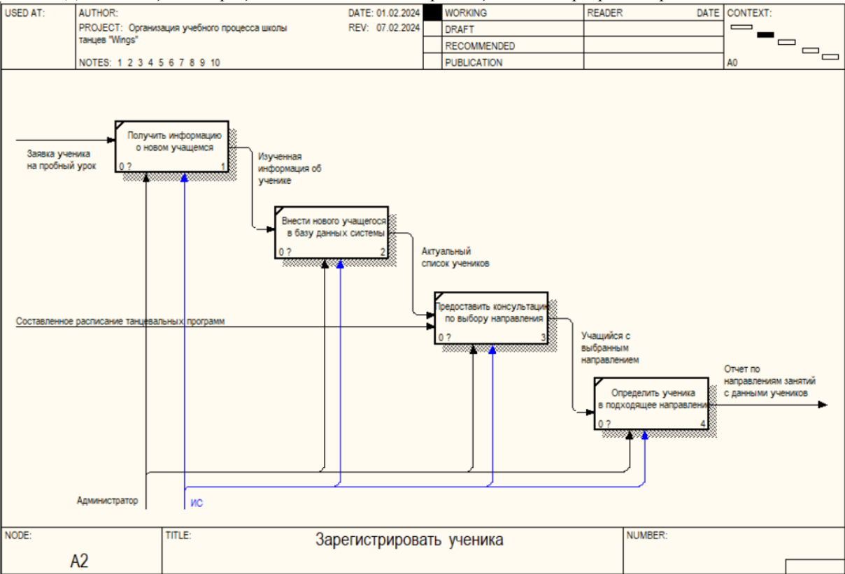
Рис.6. Декомпозиция подпроцесса «Зарегистрировать ученика»
