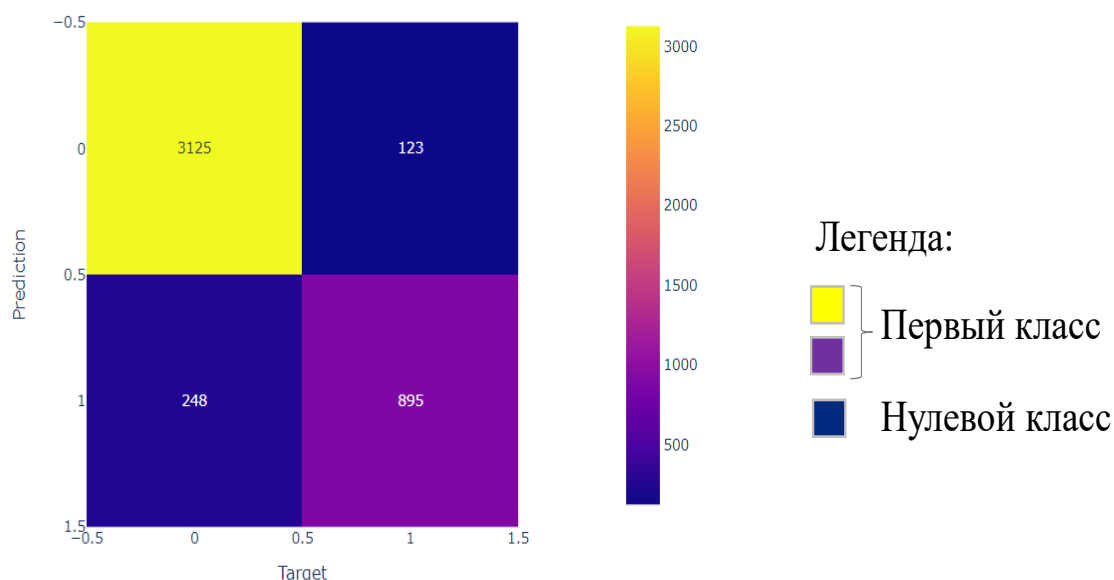
Рис.11. Модель обучения логистической регрессии
