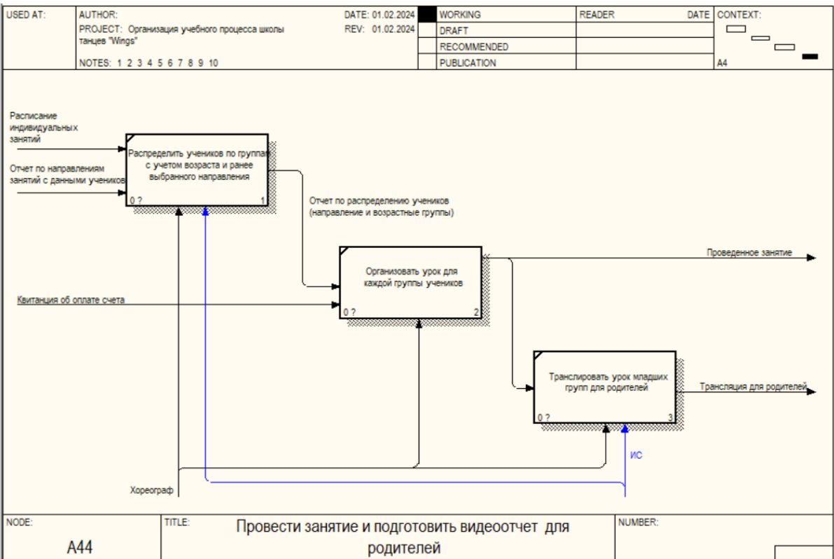
Рис.9. Декомпозиция подпроцесса «Провести занятие и подготовить видеоотчет для родителей»
